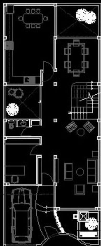
Primera Planta
