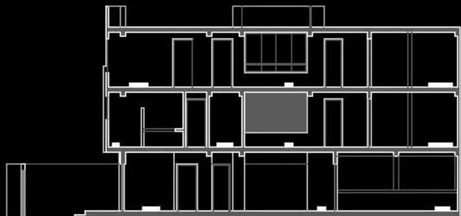
Corte B-B
